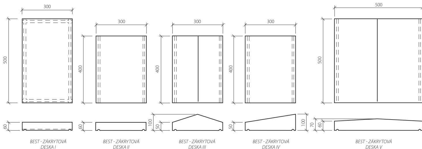
detail okapničky BEST - ZÁKRYTOVÁ DESKA I - V
